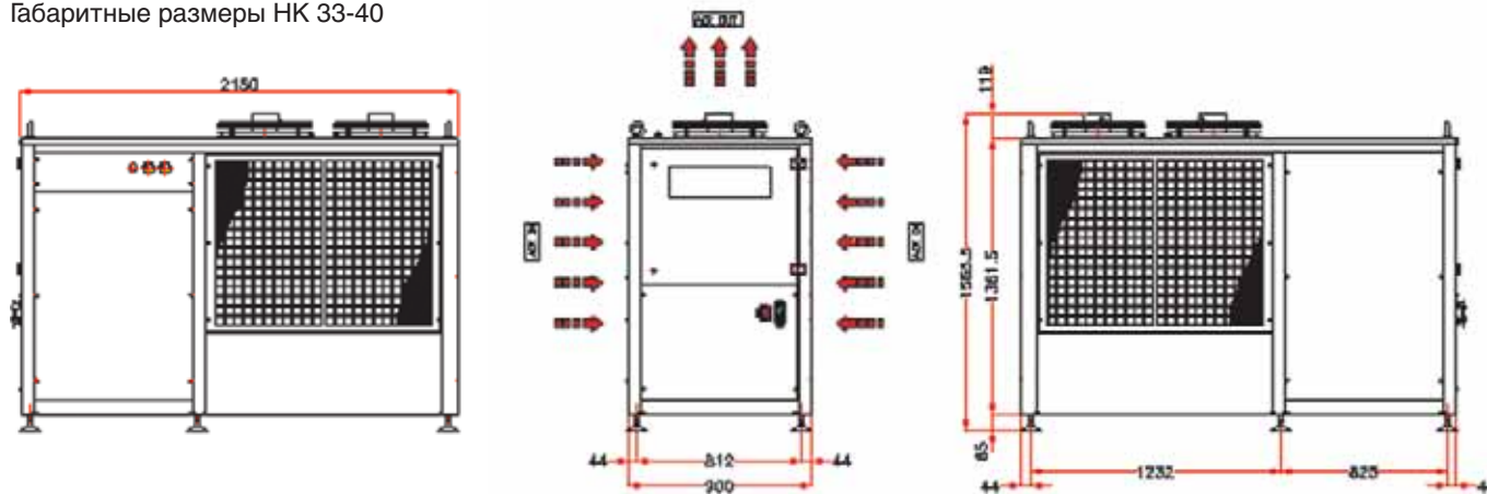
Габаритные размеры НК 33-40
