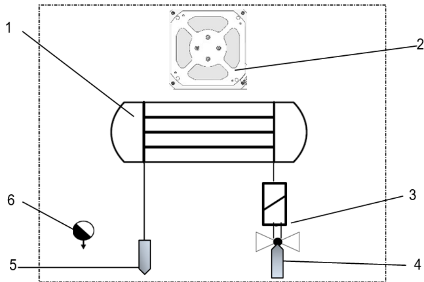
Рис. 3 - Холодильный контур
