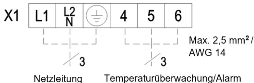
Abbildung 11 – Elektrischer Anschluss
