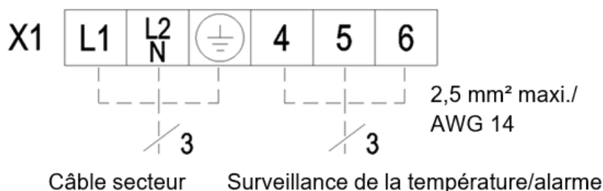
Illustration 11 – Branchement électrique
