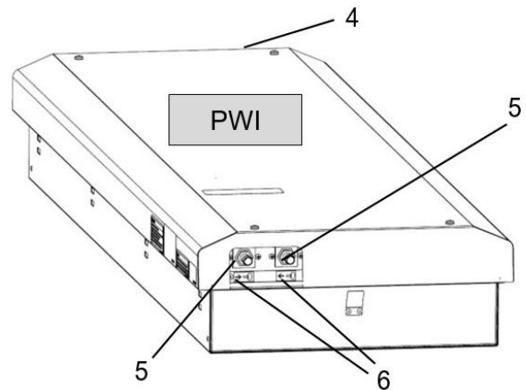
Immagine 9 - Collegamenti dell'acqua di raffreddamento Boccole filettate per tubo flessibile (vista dall'alto)
