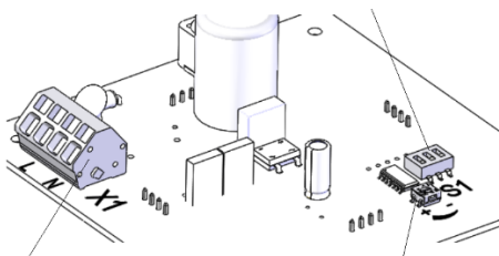
X1 Steuerung der Betriebsspannungsan- Lichtintensität (15 – 100%) schluss
