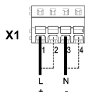
X1 Raccordement de la tension des service X2 Entrée de commande externe S1 Choix du mode opératoire S2 Commande de l'intensité lumineuse (15 - 100 %)
