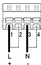
Externer Steuereingang
