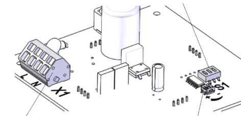
X1 Raccordement de la tension de service S1 Commande de l'intensité lumineuse (15 - 100 %)
