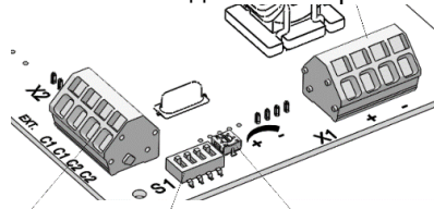
X2 Внешний управляющий вход S1 Выбор режима работы Регулирование интенсивности освещения (15 – 100%)
