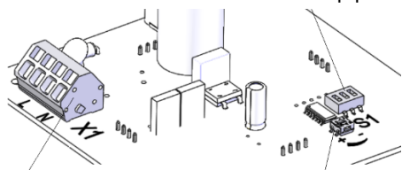
X1 Подключение рабочего напряжения Регулирование интенсивности освещения (15 – 100%)
