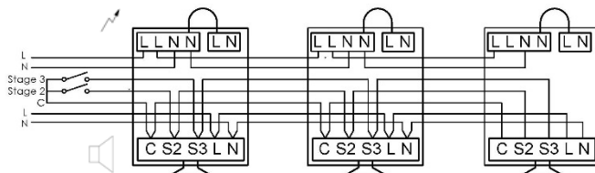
Abb. 3b. BExCS110-05D AC Vereinfachtes Blockdiagramm für separaten Betrieb
