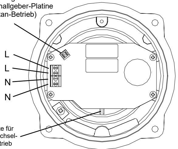
Abb. 4a Blitzleuchte AC-Version
