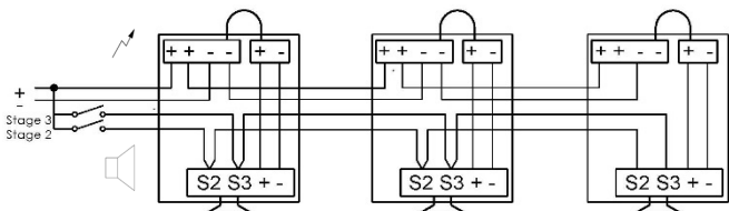
Abb. 6a. BExCS110-05D DC Vereinfachtes Blockdiagramm für Simultan-Betrieb (positive Ansteuerung)
