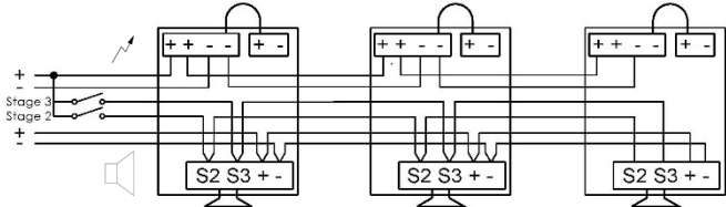
Abb. 6b. BExCS110-05D DC Vereinfachtes Blockdiagramm für separaten Betrieb (positive Ansteuerung)
