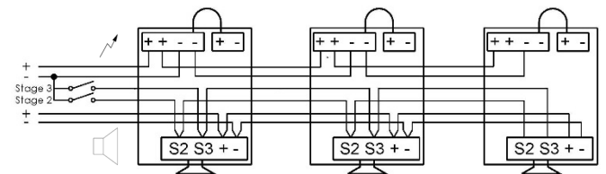
Abb. 5b. BExCS110-05D DC Vereinfachtes Blockdiagramm für separaten Betrieb (negative Ansteuerung)
