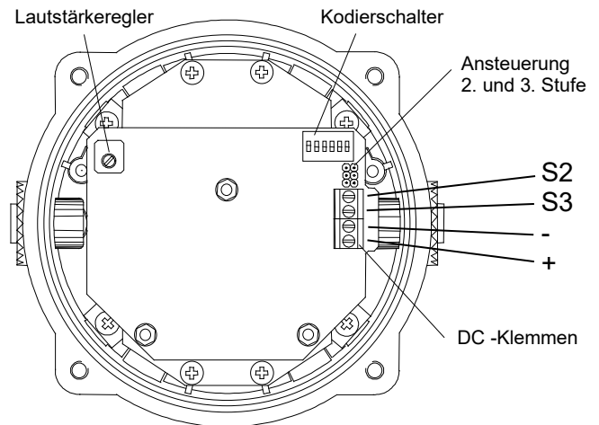
Abb. 6a Schallgeber DC-Version
