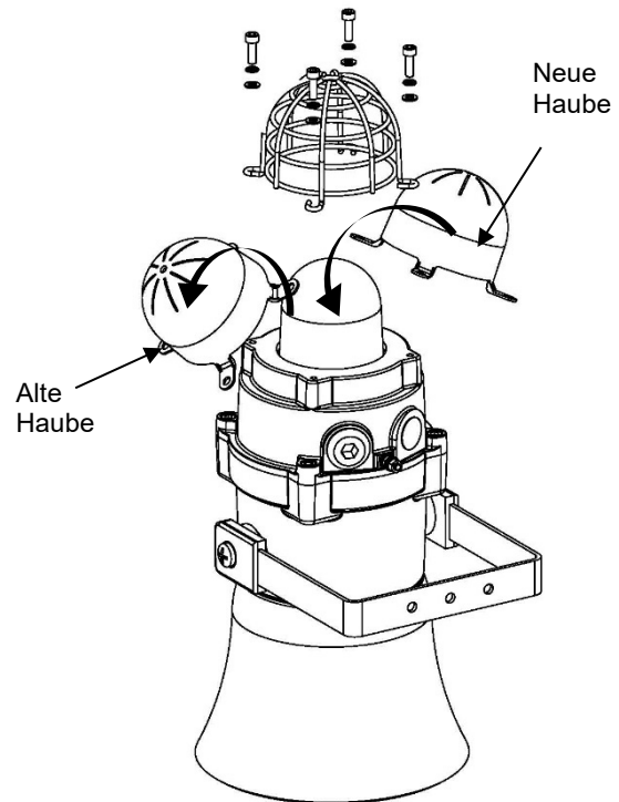
Abb. 12 Wechsel der Haube
