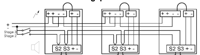
Abb. 5a. BExCS110-05D DC Vereinfachtes Blockdiagramm für Simultan-Betrieb (negative Ansteuerung)
